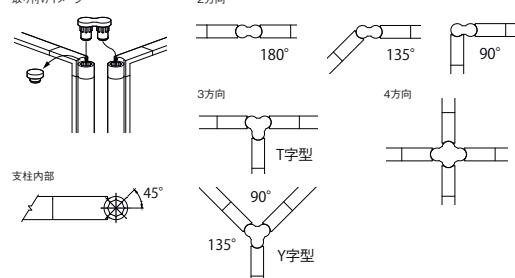
取り付けイメージ
