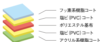
キャンバス構造概略図
